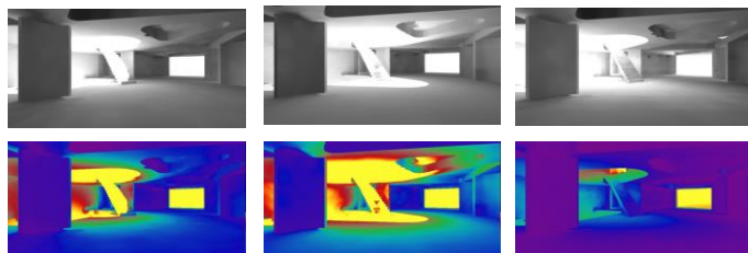
屋光の挙動をシミュレーションで把握→座席レイアウトを決定
