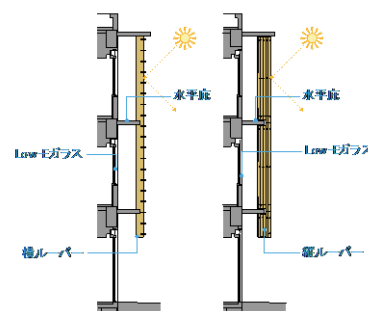
■ルーバー断面 (左：南面、右：その他方位)
