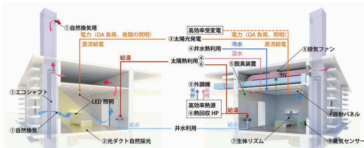
ゼロエネルギー病室 概念図
