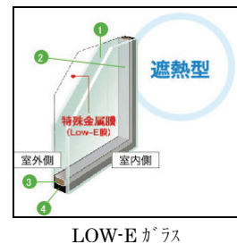
LOW-Eガラス
