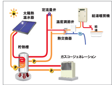
運転パターン② 日射量が少ない日(冬場)
