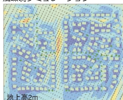
風環境シミュレーション
