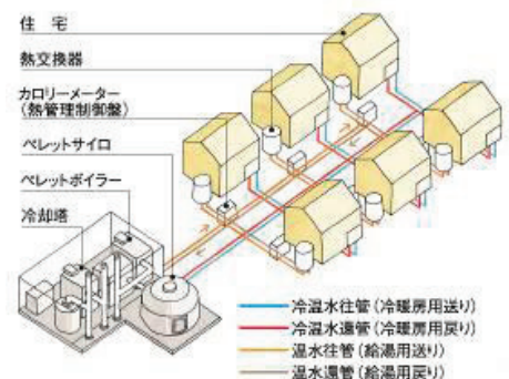
●地域集中冷暖房のシステム図
