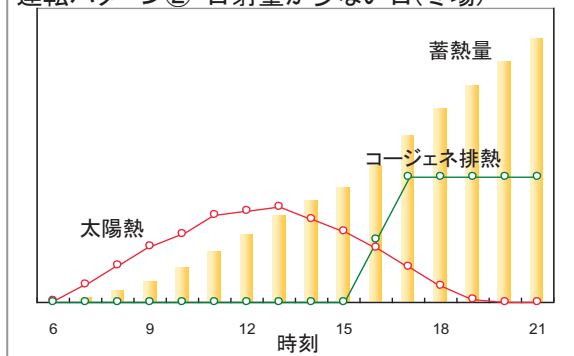
運転パターン② 日射量が少ない日(冬場)
