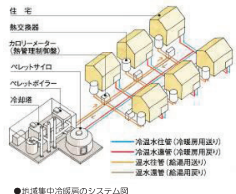
●地域集中冷暖房のシステム図
