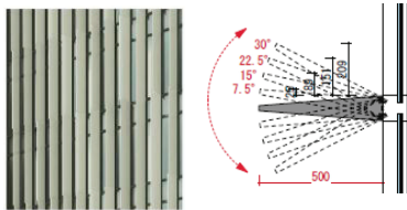
グラデーションルーバー詳細
