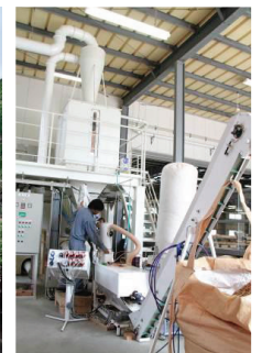
●木質ペレット製造風景
