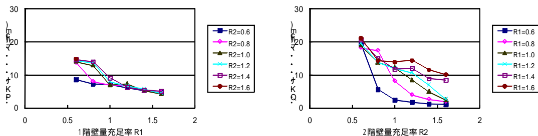
図-6.3.5 最大応答変位の計算結果 3 KiK-net 一関西 (IWTH25) EW 成分に対する応答
