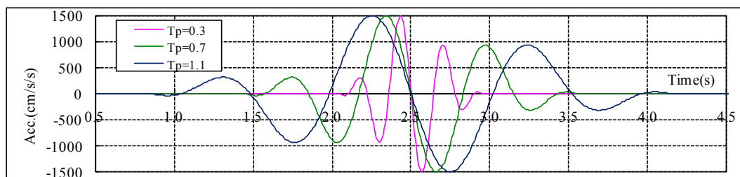
図-6.2A.1 入力波 (最大加速度 1500gal)
