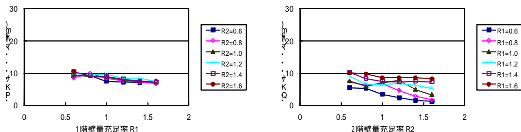
図-6.3.6 最大応答変位の計算結果 4 KiK-net 東成瀬 (AKTH04) EW 成分に対する応答
