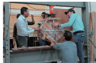
中南米地震工学コースの現地での構造実験 Structural test in El Salvador (Earthquake Engineering for Latin America Course)
