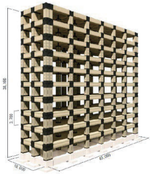
木質系パネル・集成材複合部材による10階建ての概要 Outline of 10-story building with wood panel and laminated wood composite members
