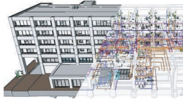
統合BIMモデルデータ（意匠、構造、設備） Integrated BIM model data (design, structure, equipment)
