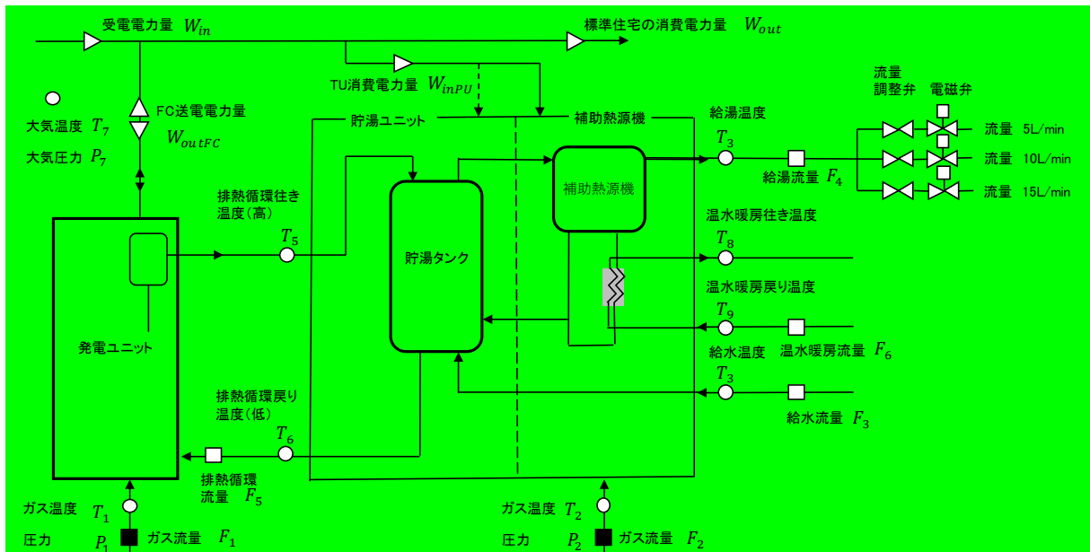
図5 試験装置及び計測ポイント(例)
