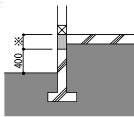
図 1 GL+400 を超える基礎等
