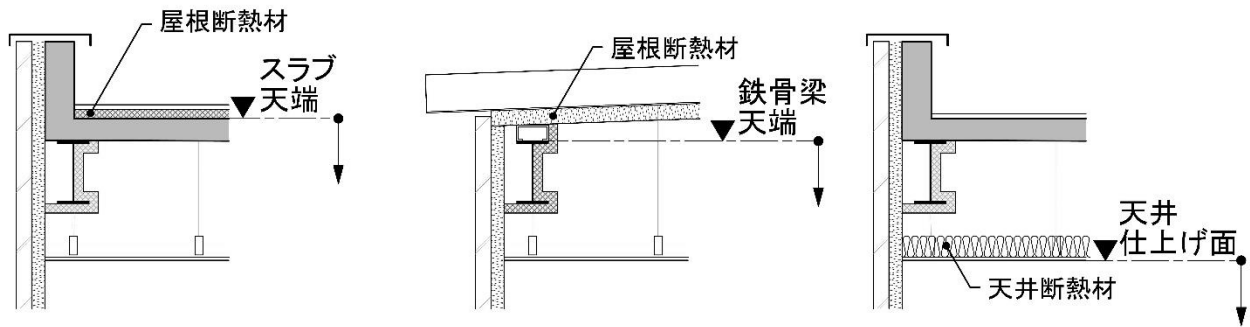
[陸屋根 屋根断熱 スラブ有りの場合]
