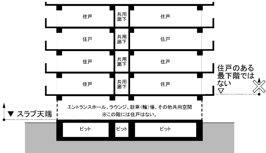
図 3.10 1階部分に住戸がない場合の例
