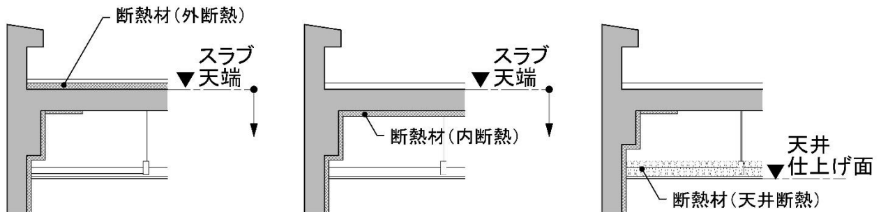
【屋根 外断熱の場合】
