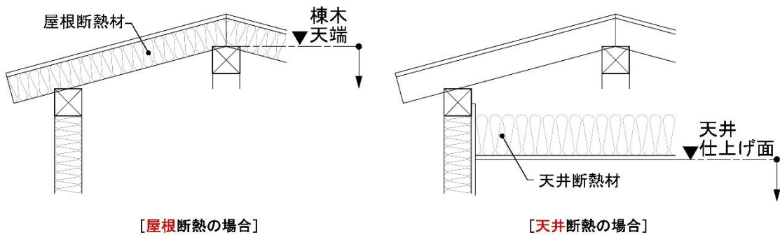
図 3.8 木造（CLT工法を除く）における上端の基点
