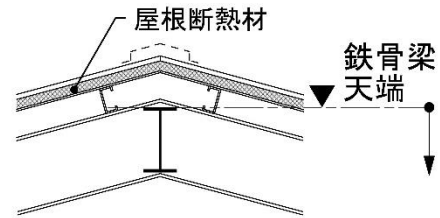
[勾配屋根 屋根断熱 スラブ無しの場合]
